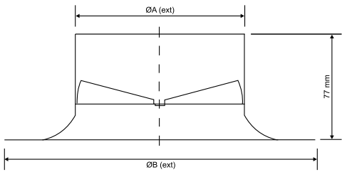
Размеры CRS
