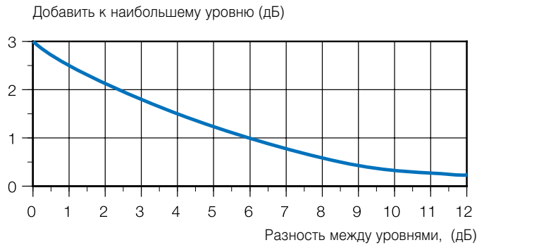
Рис. 5. Логарифмическое сложение
