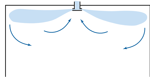
Рис. 21. Горизонтальная подача воздуха потолочным диффузором
