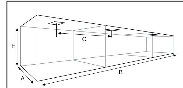
Рис. 19. Большое помещение, вентилируемое несколькими потолочными диффузорами
