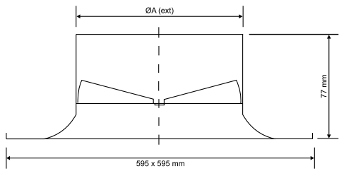
Размеры CRS-T
