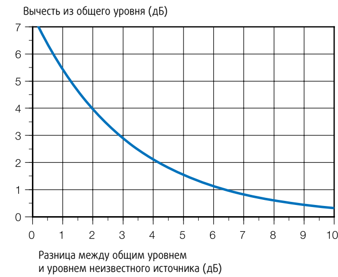
Рис. 6. Логарифмическое вычитание
