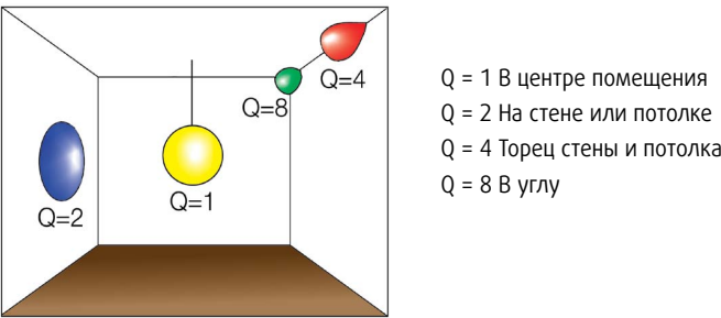
Рис. 1. Коэффициенты направленности для различно расположенных источников шума
