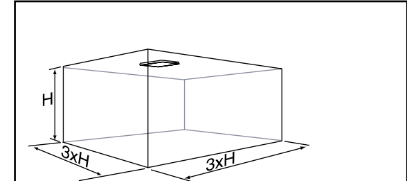
Рис. 18. Небольшое помещение, вентилируемое одним потолочным диффузором Если помещение
