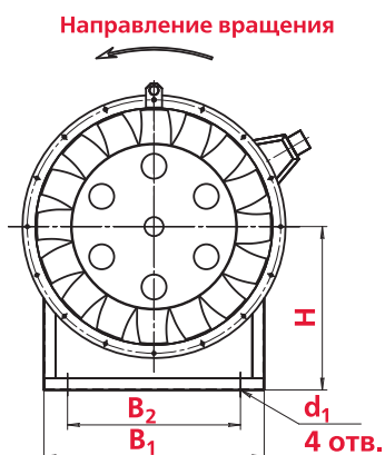
Компоновка 03
