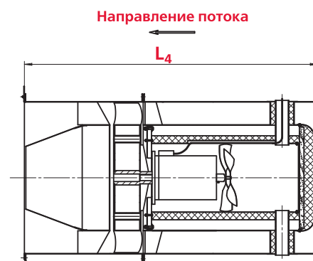
Компоновка 02
