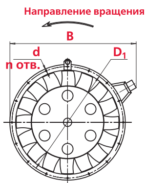
Компоновка 01
