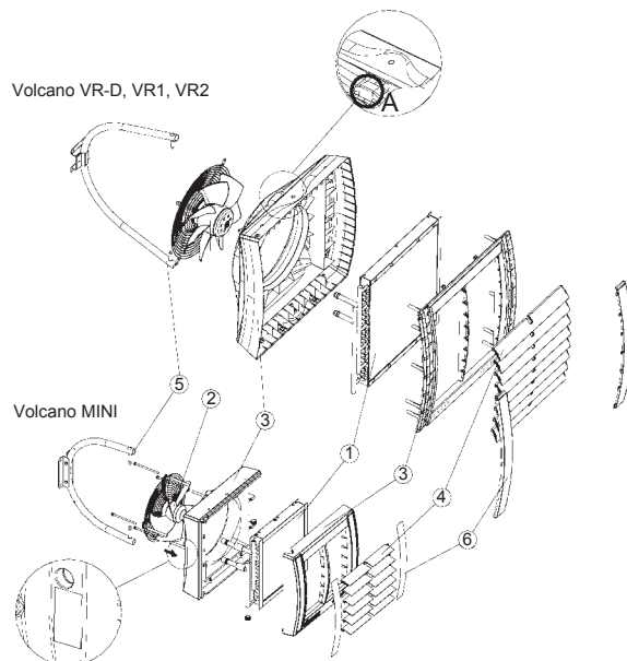
1. VÝMĚNÍK TEPLA; 2. AXIÁLNÍ VENTILÁTOR; 3. OPLÁŠTĚNÍ; 4. SMĚROVÉ LAMELY VZDUCHU; 5. PŘÍKLADOVÁ MONTÁŽNÍ KONZOLE; 6. BOČNÍ LIŠTY; A. DATOVÝ ŠTÍTEK
